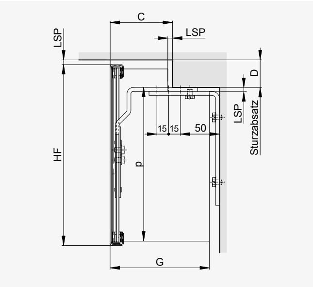
1.3 Gerade Abdeckung.
