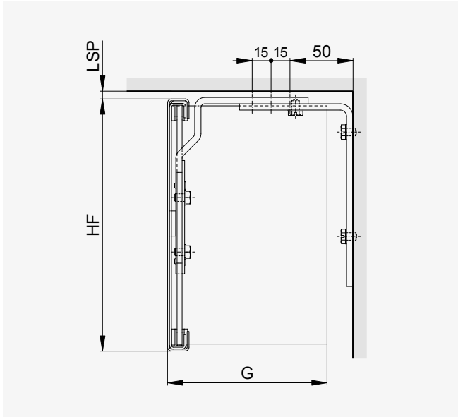
1.1 Gerade Abdeckung.
